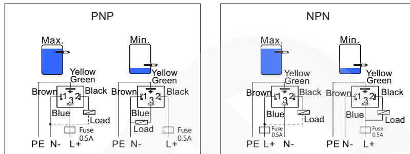
DIN Cable Wiring Diagram
