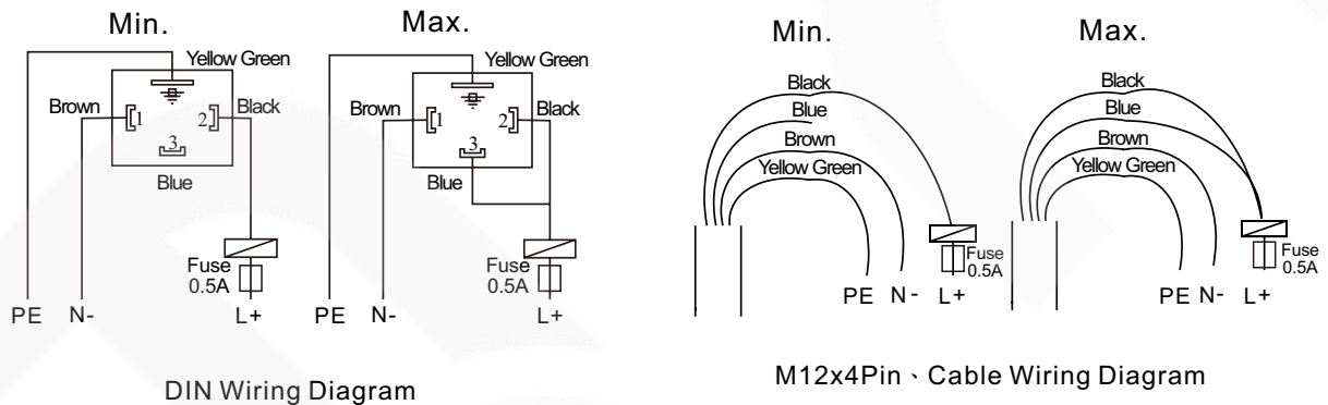
DIN Wiring Diagram
